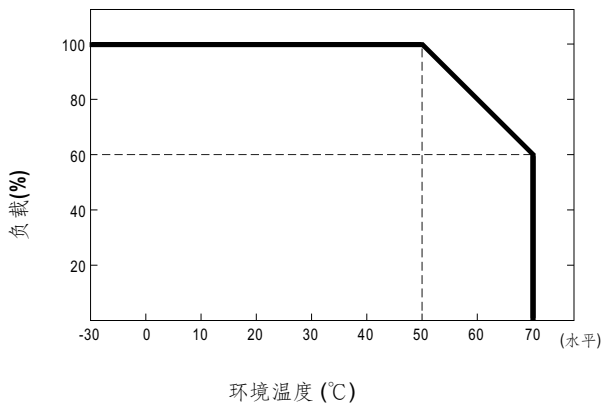
■ 减额曲线
