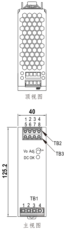
主视图
